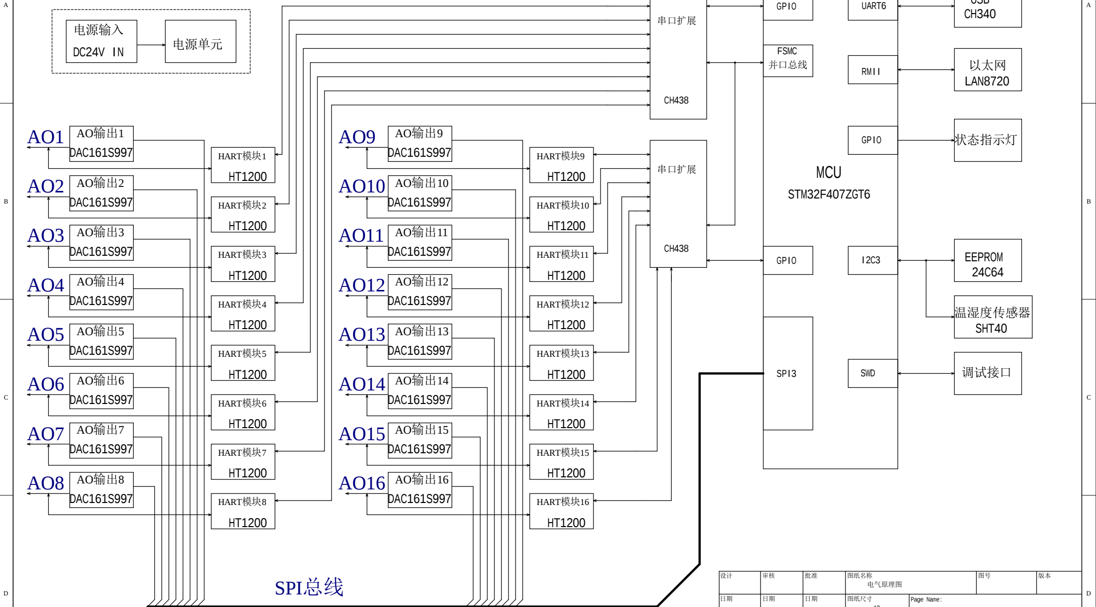
I_Valve_Debugging_V100 系统框图
