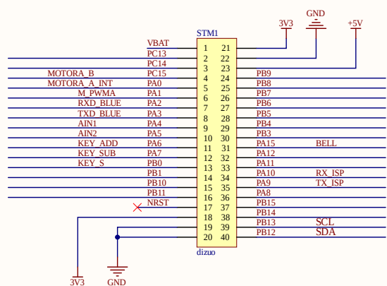
STM32F103C8T6 主控
