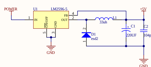
+12V 转5V0
